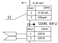
Схема соединения БИ и БПВС
